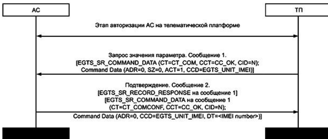
Рисунок 76 - Запрос значения параметра
